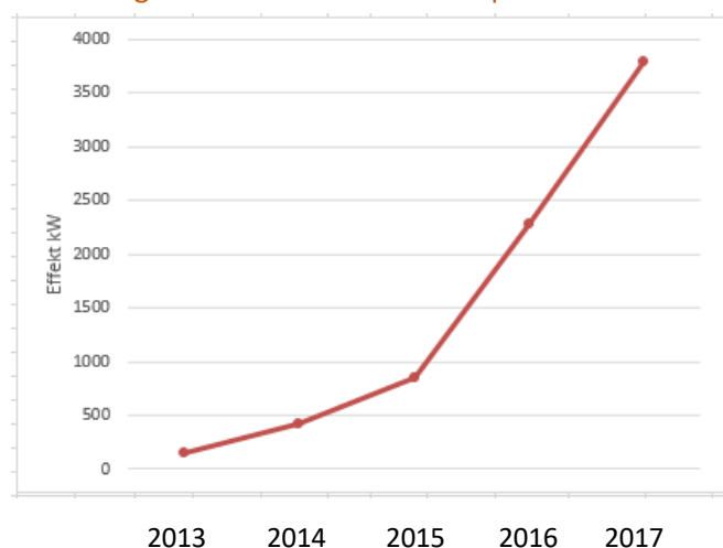
Utveckling av installerad effekt solel på Gotland
